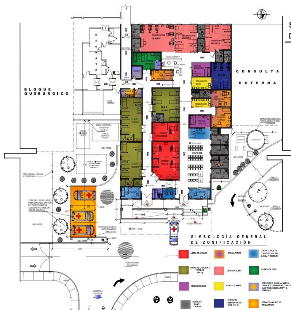
PLANTA DE DISTRIBUCIÓN ZONIFICADA PROPUESTA PARA LA EMERGENCIA A REEMPLAZAR
