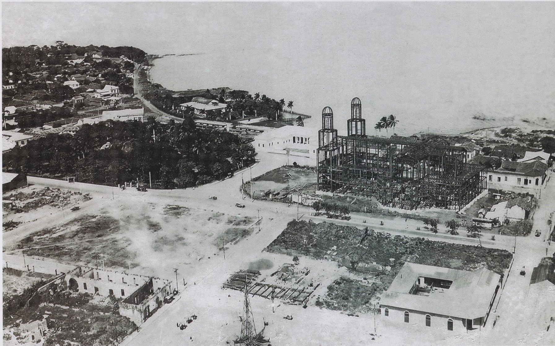
No. 128_Vista aérea de Managua. Observe la Catedral en construcción con su armazón de hierro [c. 1933] Aerial view of Managua. Note the Cathedral under construction, its iron framework completed
